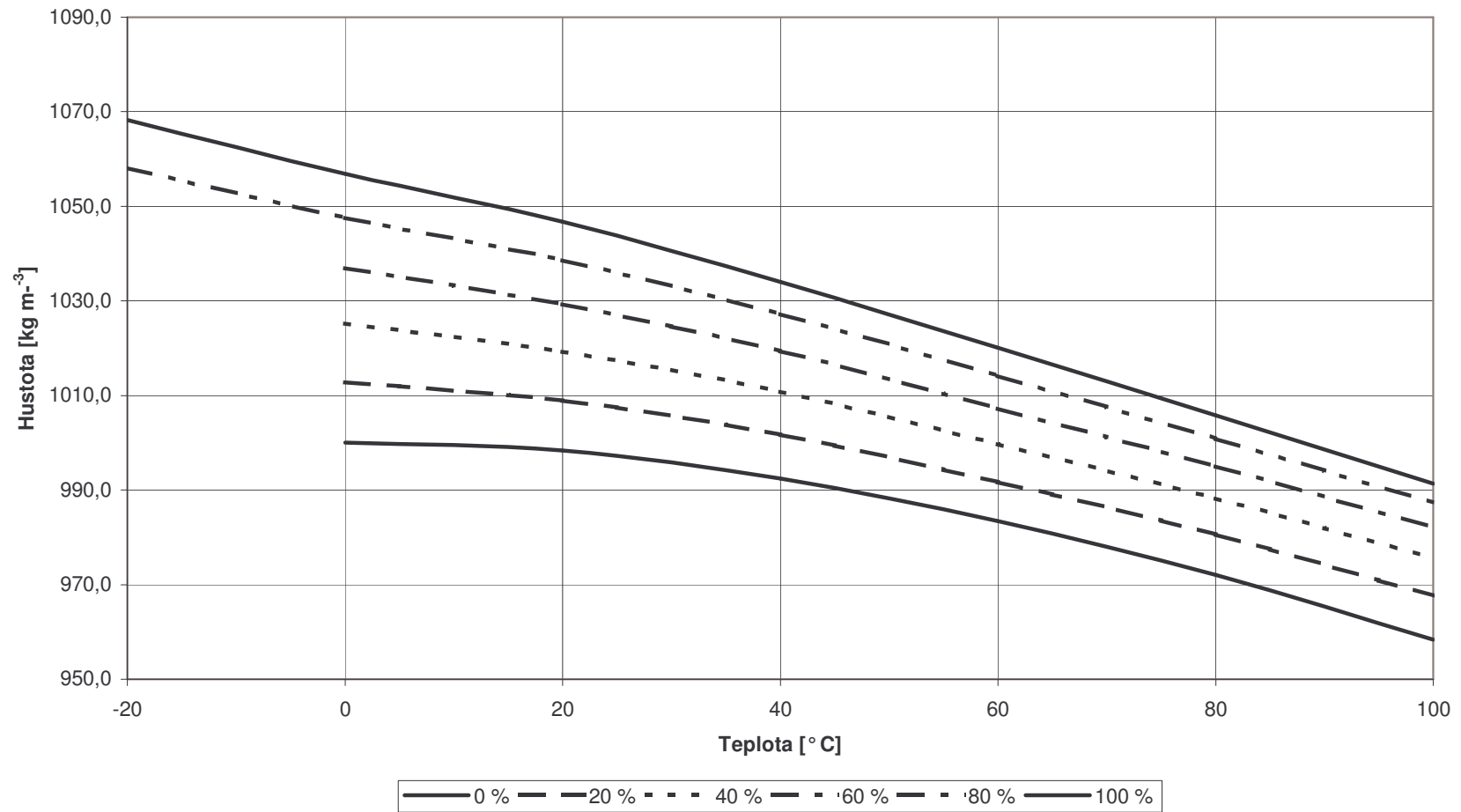
Závislost hustoty na teplotě pro různé koncentrace Solarenu
