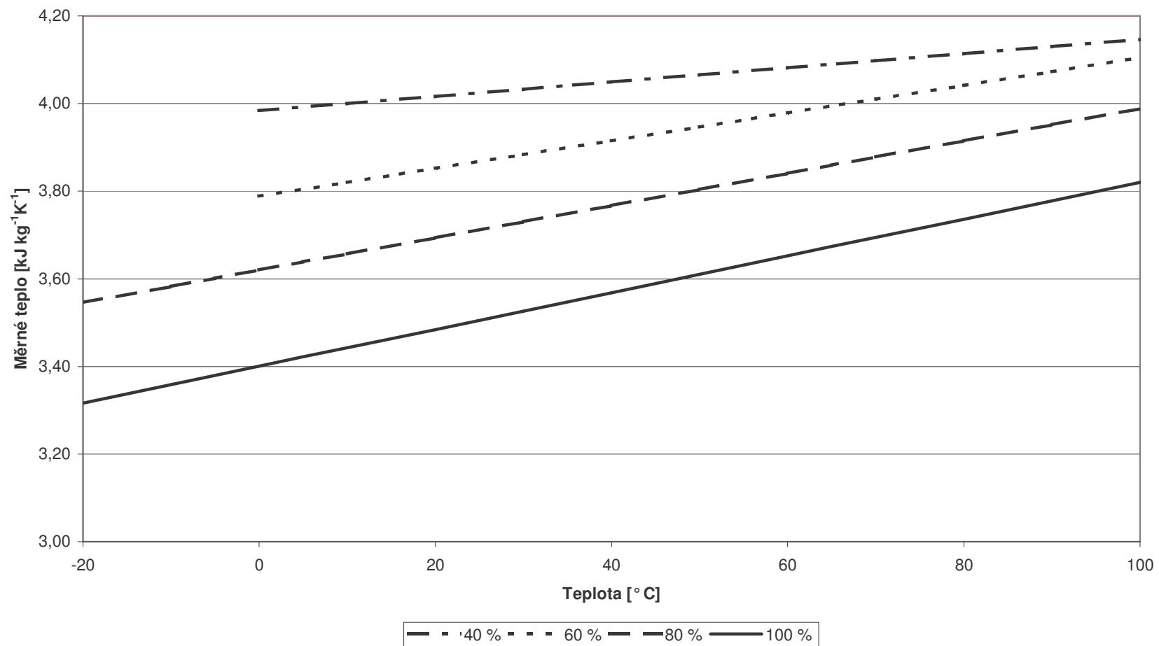
Závislost měrného tepla na teplotě pro různé koncentrace Solarenu
