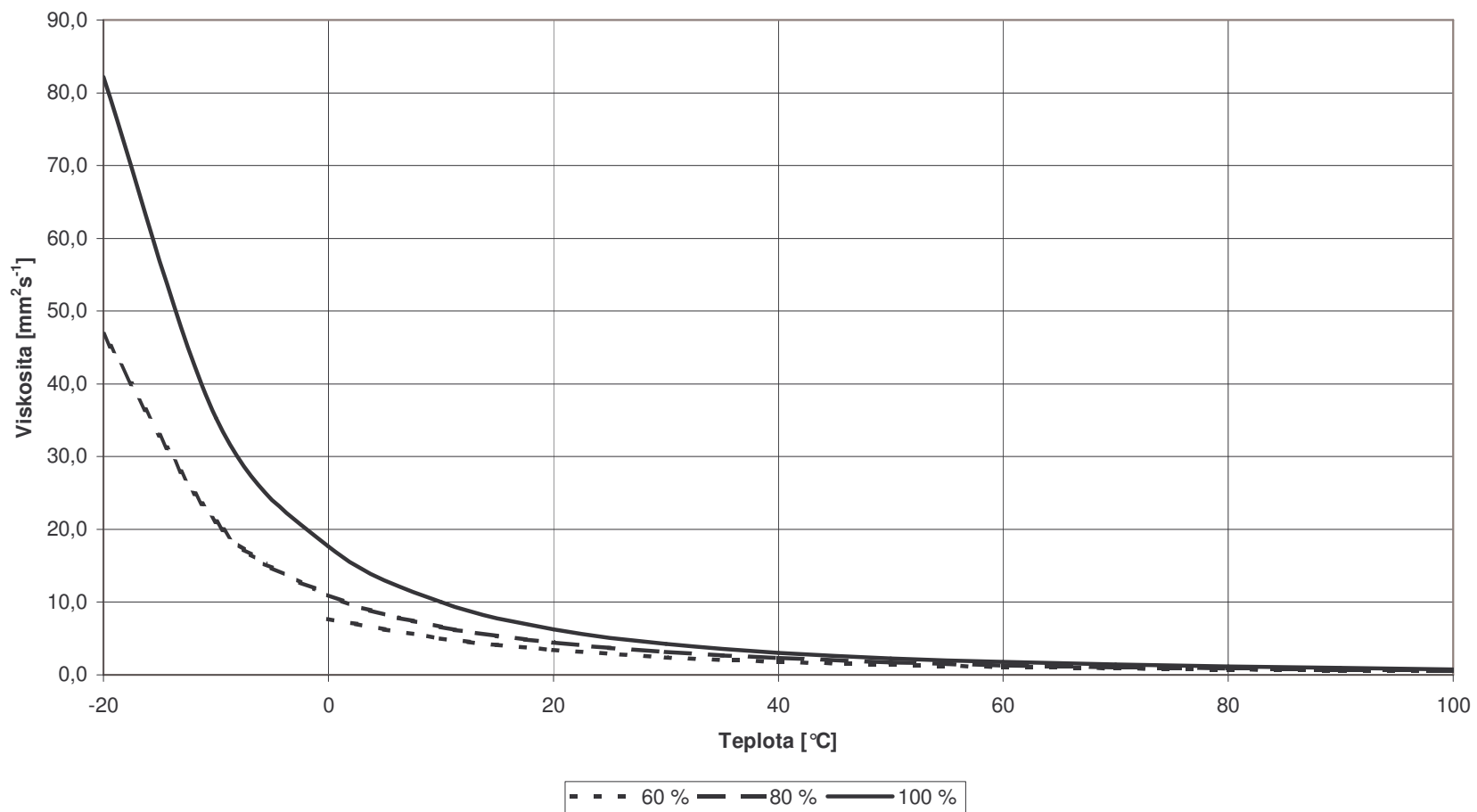
Závislost viskozity na teplotě pro různé koncentrace Solarenu
