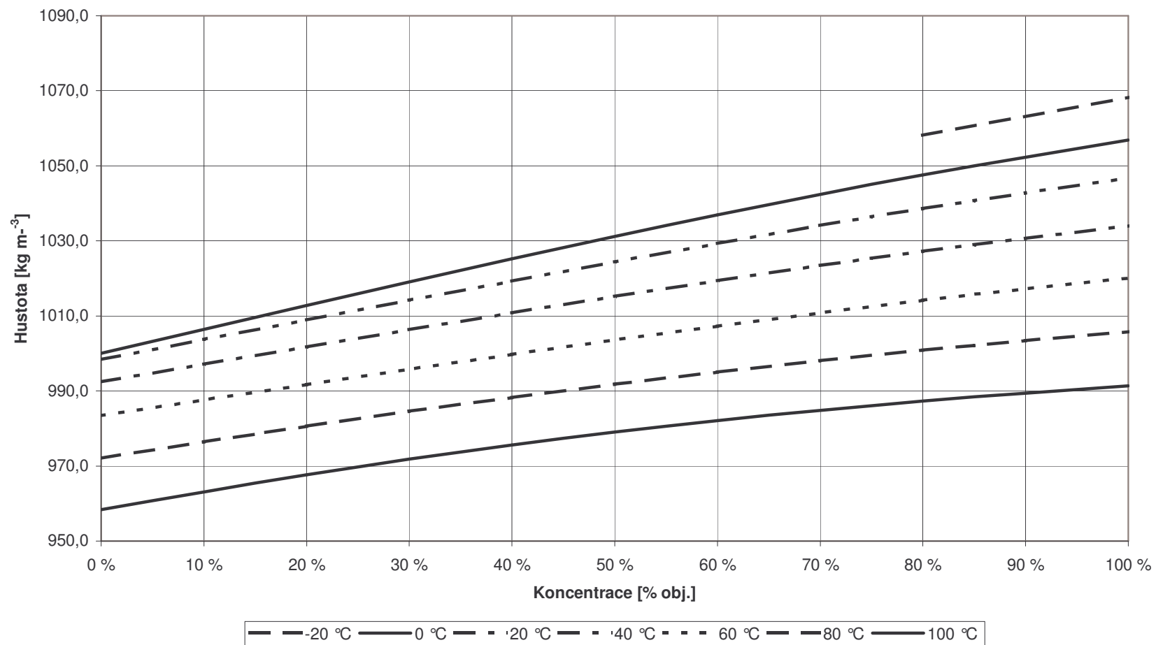
Závislost hustoty na koncentraci Solarenu pro různé teploty
