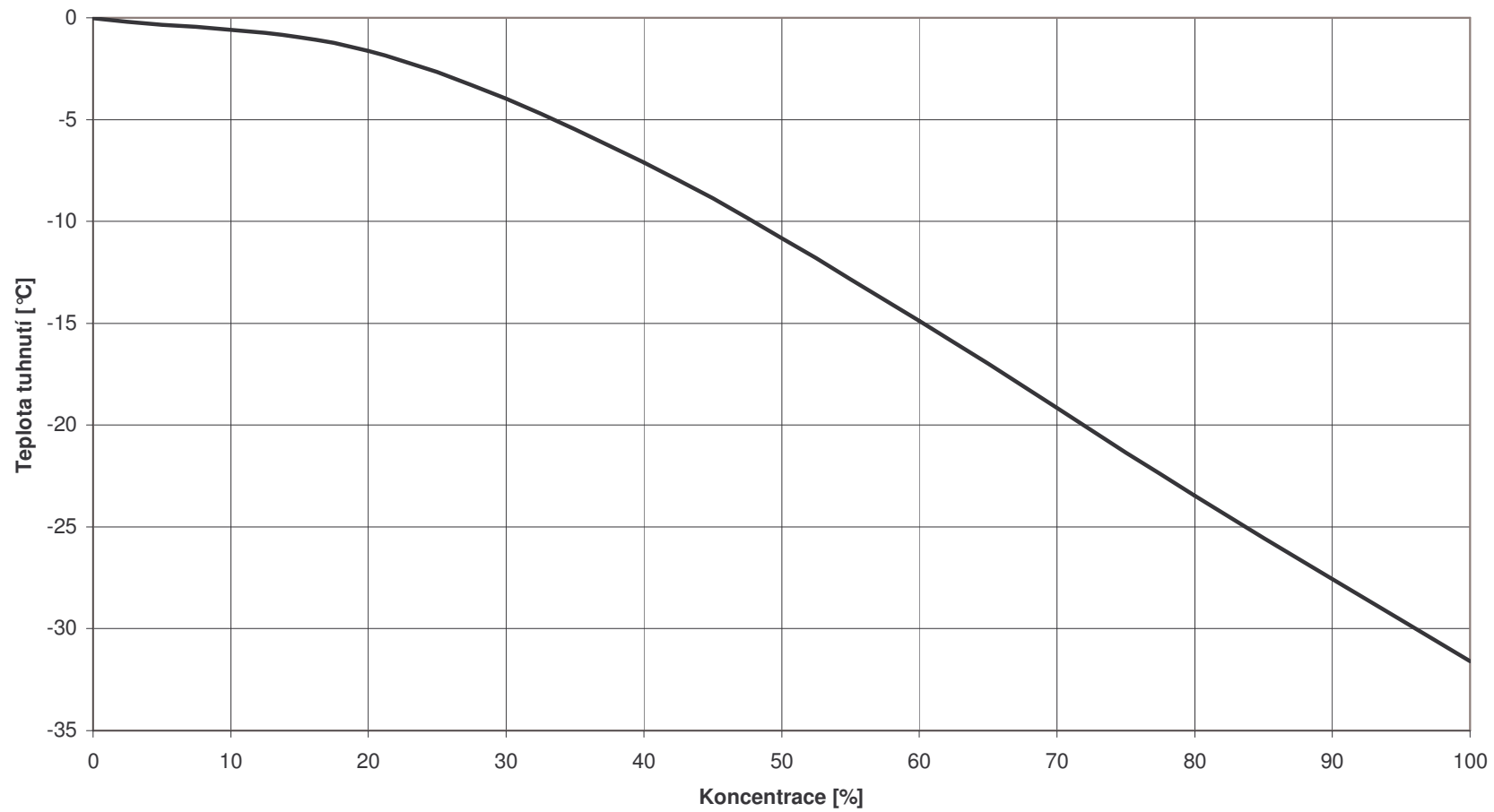
Závislost teploty tuhnutí Solarenu na objemové koncentraci
