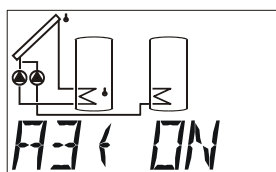
A3 aktivní (jako výstup spín. hodin)
