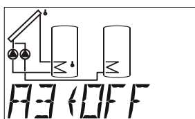
A3 deaktivováno
