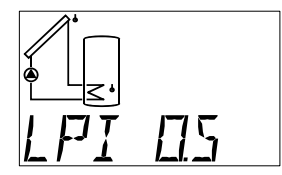
Litr na jeden impuls Zobrazení jen, pokud S6 = VSG
